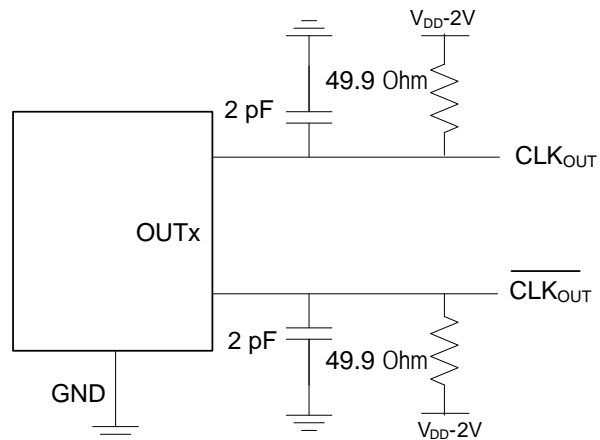
LVPECL
