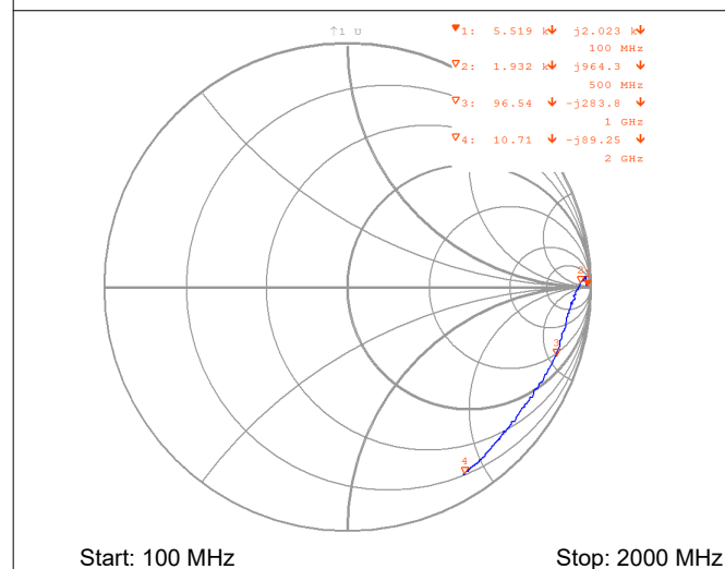
Figure 6-10. Fin Input Impedance
